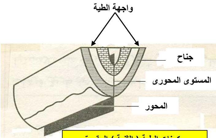
مكونات الطية (الثنية) المقعرة
