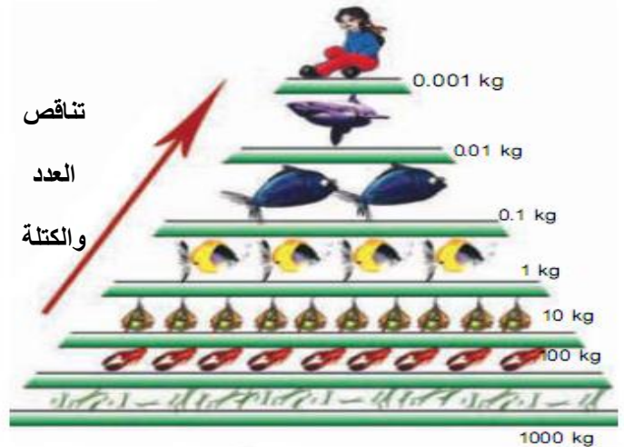
هرم الطاقة البحرى (رسم مستويات سلسلة الغذاء البحرى)
