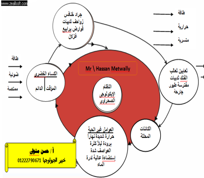
كوكب الأرض / الغلاف الحيوى وعلاقته بالأغلفة الأخرى
