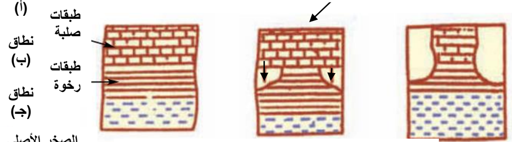
النحت المتباين وتأثير الجاذبية (تكوين المصطبة)
