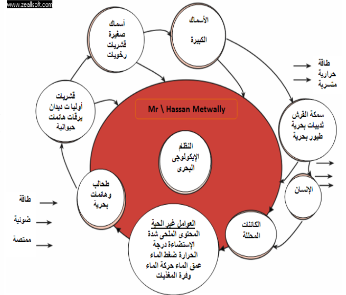
نموذج لكائنات ومكونات النظام الايكولوجى، وعلاقتها بسريان الطاقة ودوران المواد
