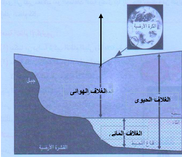
كوكب الأرض / الغلاف الحيوى وعلاقته بالأغلفة الأخرى
